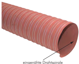
eingenähte Drahtspirale
