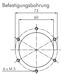
Befestigungsbohrung
