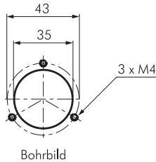
Bohrbild
