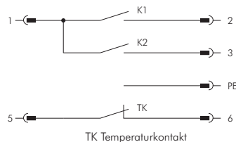
TK Temperaturkontakt
