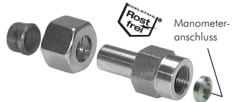
Dichtkantenringe als Ersatzteil auf Seite 911
