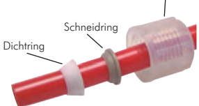
Anschlussprinzip „2“
